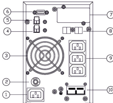
ИБП 1 кВА
